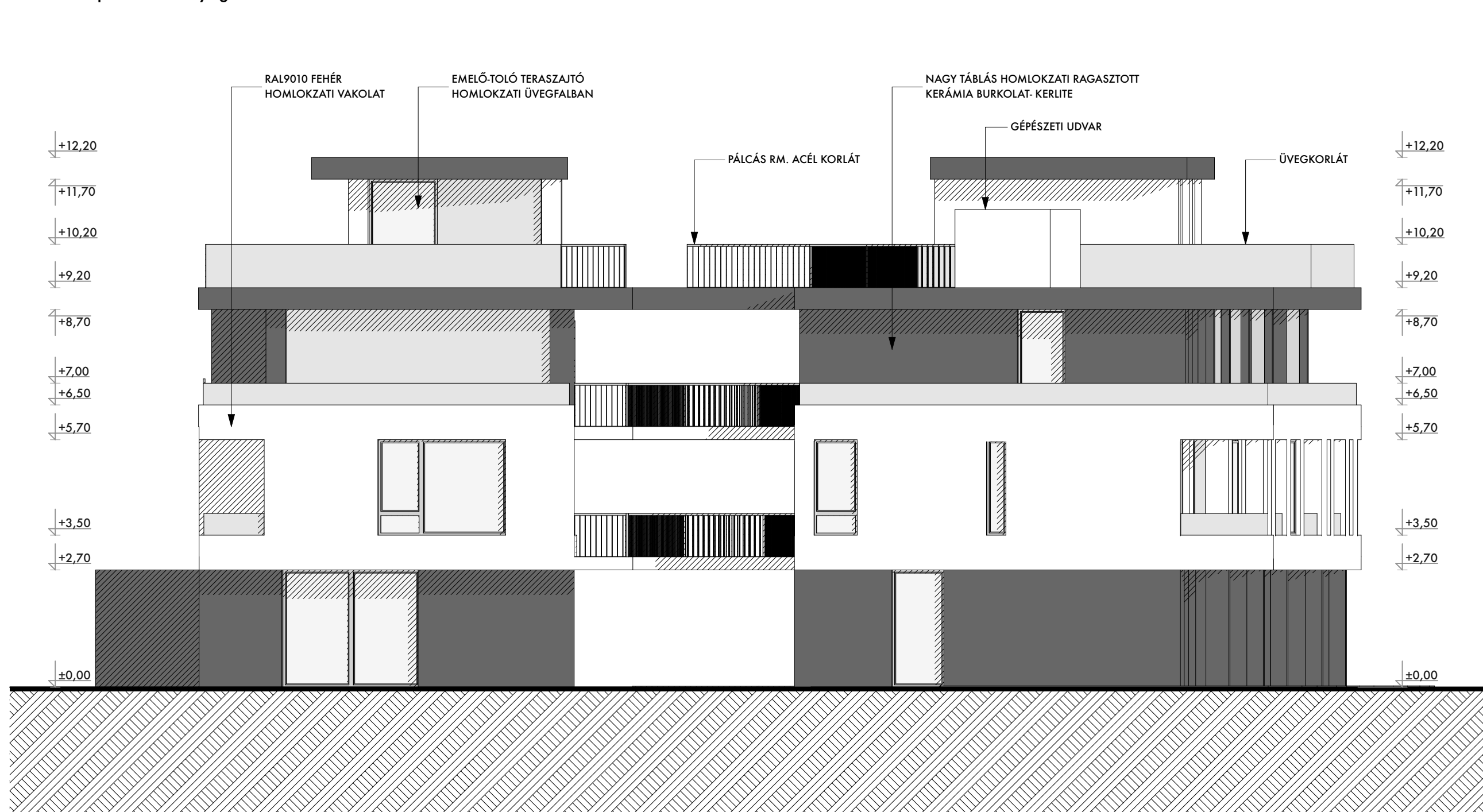
"A" épület észak-nyugati homlokzat
